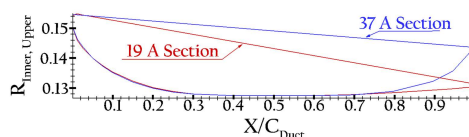
شکل ۱۲- مقطع مجرا استاندارد ۱۹ آ و ۳۷ آ [۱]
