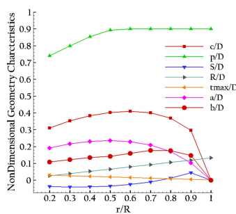
شکل ۳- مشخصات هندسی پروانه
