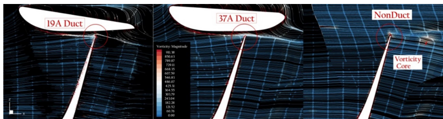
شکل ۱۶- خطوط جریان با ۱۸۰۰ بردار، رنگ‌شده به‌وسیله گردابه 1/s در ضریب پیشروی ۰/۵ و موقعیت Y=0
