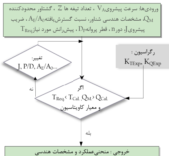
شکل ۱- روند نمای طراحی پروانه به روش سری استاندارد
