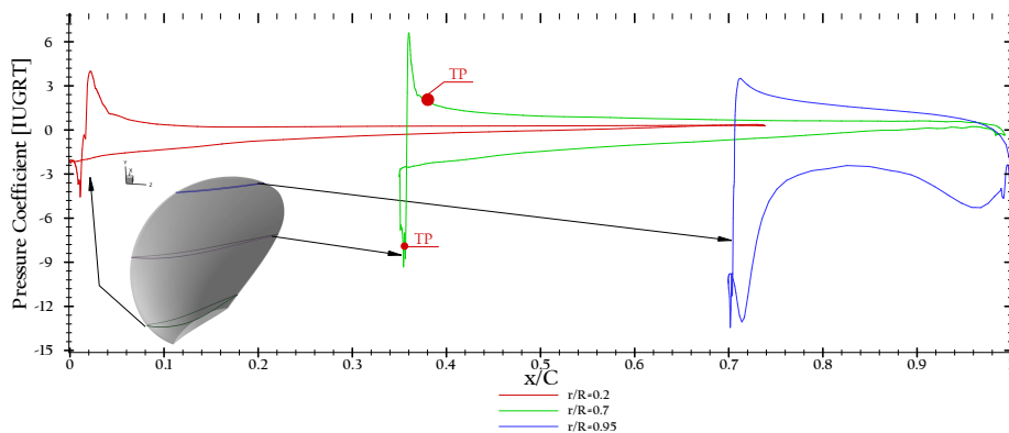
شکل ۱۱- ضریب فشار حول سطوح مکشی و فشاری پروانه در J=0.4 با مدل IUGRT
