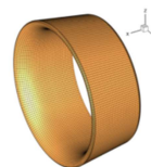
شکل ۱۳- شبکه‌بندی سطحی روی مجرا استاندارد ۱۹ آ
