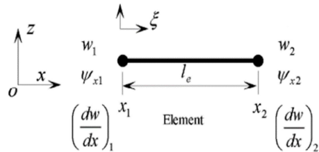
شکل ۲- المان دو گره‌ای میکرو تیر پیزوالکتریک
