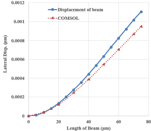
شکل ۶- تغییر مکان عرضی تیر در نرم‌افزار Com Sol با کدنویسی المان محدود
