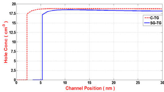
شکل ۷: غلظت حفره‌ها در راستای Y
