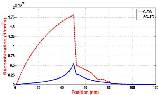
شکل ۸: باز ترکیب برای دو ساختار SG-TG و C-TG
