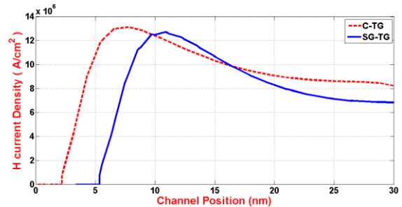
شکل ۵: چگالی جریان حفره‌ها در راستای Y
