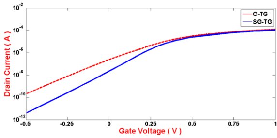
شکل ۱۲: جریان خاموشی ساختارهای C-TG و SG-TG در V_D=0/\Delta V
