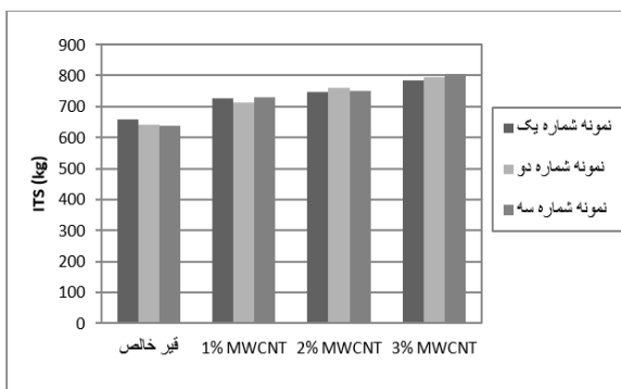
شکل ۶- مقاومت کشش غیر مستقیم نمونه‌های حاوی قیر خالص و اصلاح شده با نانولوله کربنی در حالت خشک با مصالح سیلیسی
