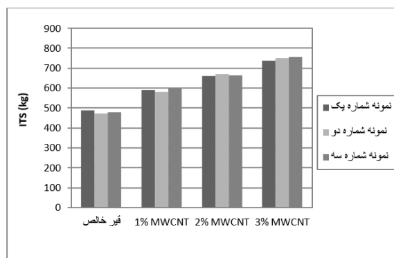
شکل ۸- مقاومت کشش غیر مستقیم نمونه‌های حاوی قیر خالص و اصلاح شده با نانولوله کربنی در حالت اشباع با مصالح سیلیسی
