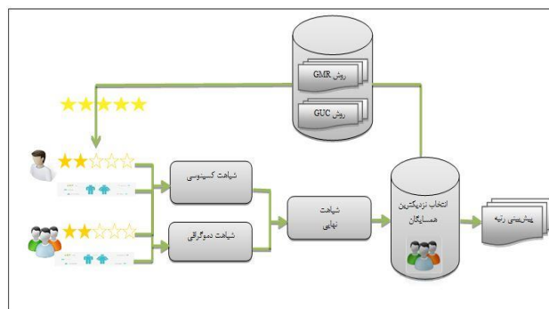
شکل ۱: چارچوب کلی روش پیشنهادی.
