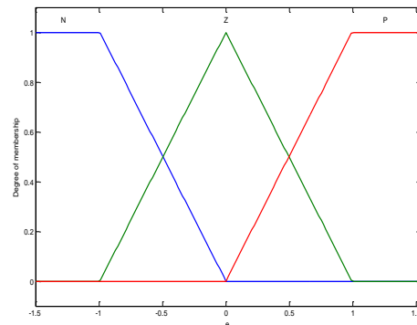
شکل ۷: توابع تعلق تنظیم شده برای e
