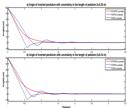
شکل ۱۷: (a) زاویه پاندول به‌ازای افزایش ۲ برابری، (b) زاویه پاندول به‌ازای کاهش ۱/۵ برابری در طول پاندول در حضور کنترل کننده‌های FOPID و FOFPID .PFOFPID
