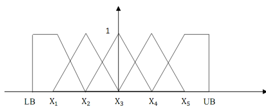
شکل 5: توابع تعلق در نظر گرفته شده برای سیستم
