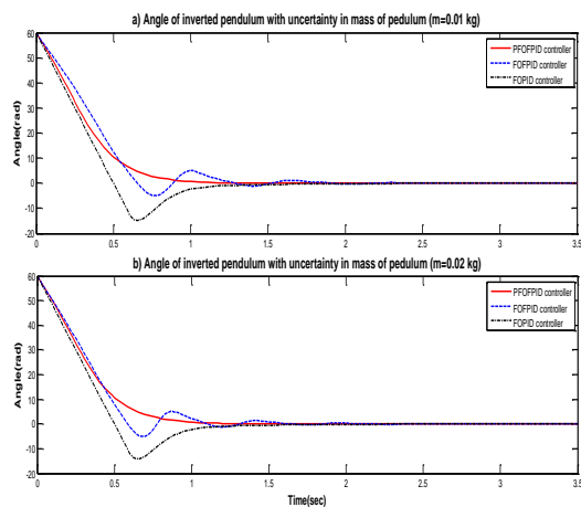
شکل ۱۳: (a) زاویه پاندول به ازای کاهش ۱۰ برابری، (b) زاویه پاندول به ازای کاهش ۵ برابری در جرم پاندول در حضور کنترل کننده‌های FOPID و FOFPID، PFOFPID
