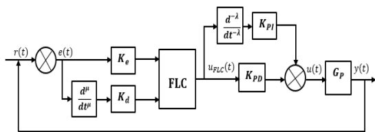
شکل ۱: بلوک دیگرام کنترل کننده FOFPID [۷]
