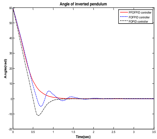
شکل ۱۰: زاویه پاندول نسبت به محور عمود در حضور کنترل کننده‌های PFOFPID، FOFPID و FOPID
