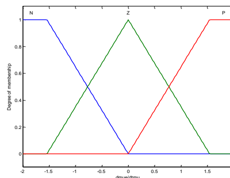
شکل ۸: توابع تعلق تنظیم شده برای \frac{d^\mu e(t)}{dt^\mu}
