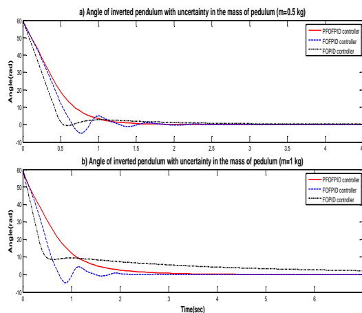
شکل ۱۴: (a) زاویه پاندول به ازای افزایش ۵ برابری، (b) زاویه پاندول به ازای افزایش ۱۰ برابری در جرم پاندول در حضور کنترل کننده‌های FOPID و FOFPID، PFOFPID
