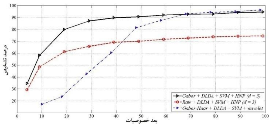
شکل ۷: نمودار مقایسه‌ای روش پیشنهادی برای مقایسه تأثیر تبدیل گابور-هار
