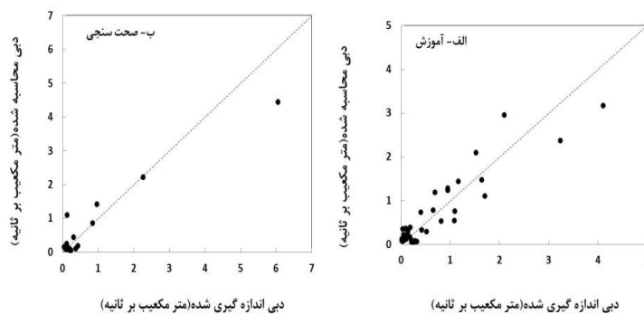
شکل (۳) پراکنش بین دبی‌های مشاهده‌ای و شبیه‌سازی شده با استفاده از مدل Wetspa. الف- مرحله واسنجی، ب- مرحله صحت‌سنجی
