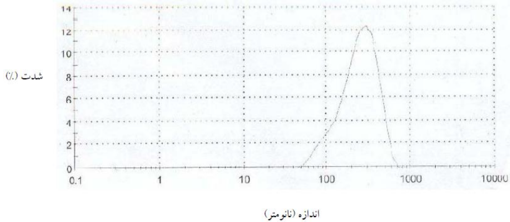
شکل ۱- توزیع اندازه (Size) نانوذرات لیپیدی جامد (نانومتر) بر اساس شاخص شدت (Intensity) فرمولاسیون تهیه شده با ۰.۵٪ لیپید (گلیسرین منواستئارات و پرسیرول) و ۲/۵٪ سورفکتانت (توئین ۸۰ و پولوکسامر ۱۸۸).
