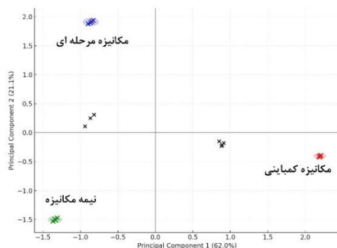
شکل ۳- پراکنش و جداسازی تیمارها بر اساس مؤلفه‌های اصلی.
