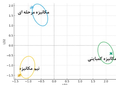
شکل ۴- مرزبندی و تفکیک تیمارها بر اساس توابع تمییز.
