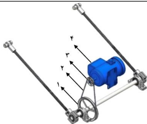
شکل ۷- سیستم انتقال توان از الکتروموتور به شاسی ارتعاشی (شامل: ۱- پولی متحرک ۲- تسمه ۳- پولی محرک ۴- الکتروموتور)
