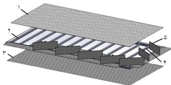
شکل ۳- اجزای سیستم الک جداکننده ثقلی
