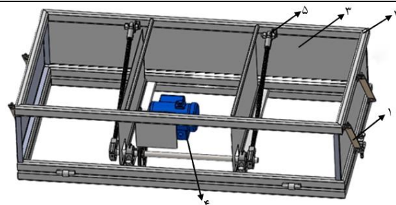
شکل ۴- واحد ارتعاشی الک (۱- فنرهای ورق ۲- شاسی ۳- ورق‌های فولادی ۴- الکتروموتور ۵- یاتاقان‌های مفصلی)
