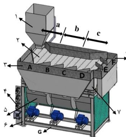
شکل ۱- طرح کلی ماشین جداکننده ثقلی
