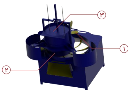
شکل ۲- دستگاه مالش ده کیلویی طراحی شده با سالیدورک (۱. لنگی ۲. استوانه بارگیری چای ۳. صفحه فشار روی چای)
