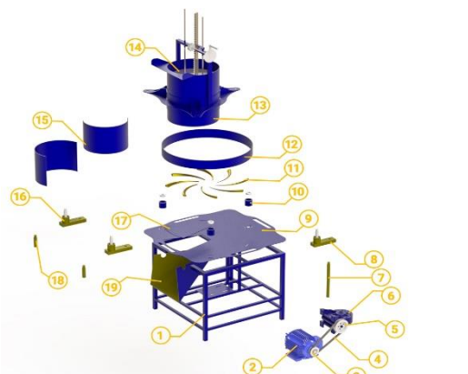
شکل ۴- طراحی انفجاری دستگاه مالش چای
