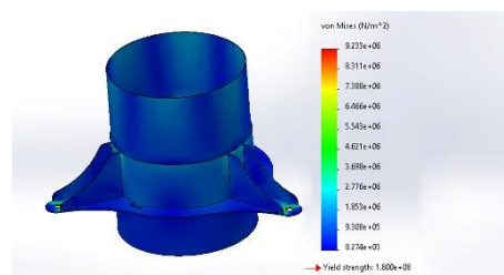
شکل ۵- تحلیل میزان تنش تسلیم به کمک نرم افزار آباکوس
