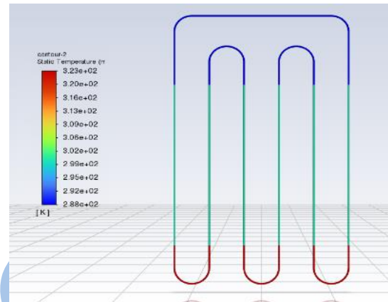
شکل ۲۶- کانتر توزیع دما در طول لوله در زمان ۰ ثانیه
