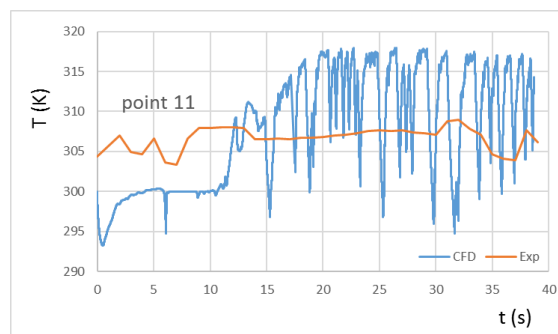
شکل ۲۲- دمای نقطه ۱۱ بر حسب زمان برای نتایج تجربی و عملی
