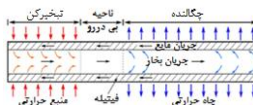
شکل ۱- ساختار لوله گرمائی ساده
