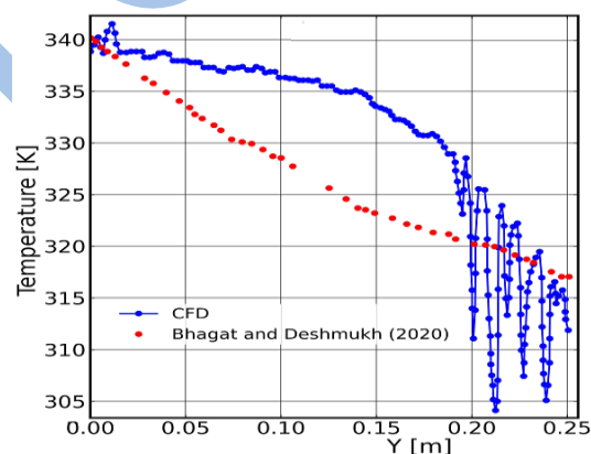
شکل ۱۶- نمودار توزیع دما در طول لوله ۱
