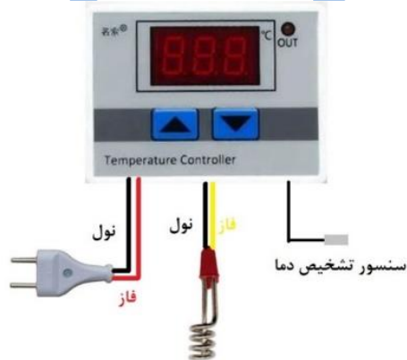
شکل ۸- مدار برق کنترلگر دما
