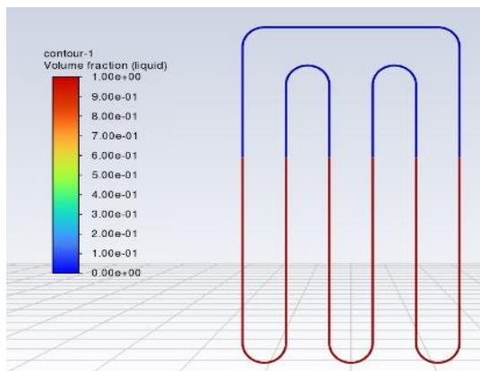
شکل ۲۳- کانتور کسر حجمی فاز مایع در زمان ۰ ثانیه
