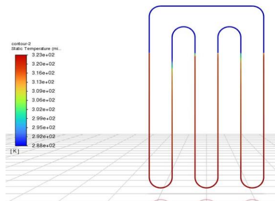
شکل ۲۸- کانتر توزیع دما در طول لوله در زمان ۳۸/۷۱۳۵ ثانیه
