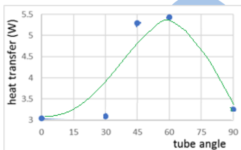
شکل ۲۹- نمودار آهنگ انتقال گرما برحسب زاویه لوله گرمایی
