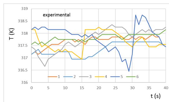
شکل ۱۲- دمای نقاط ۱ تا ۶ بر حسب زمان
