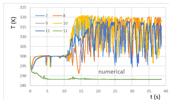
شکل ۲۰- دمای نقطه‌های ۷ تا ۱۲ بر حسب زمان
