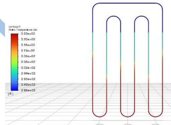
شکل ۲۷- کانتر توزیع دما در طول لوله در زمان ۲۵/۹۱۵ ثانیه
