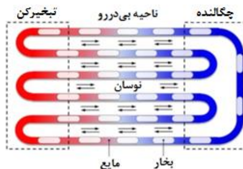
شکل ۲- لوله گرمائی نوسانی حلقه بسته
