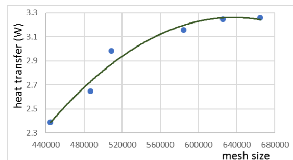
شکل ۱۵- نمودار انتقال گرما برحسب تعداد سلول‌های شبکه
