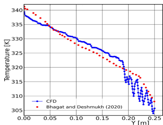
شکل ۱۷- نمودار توزیع دما در طول لوله ۲
