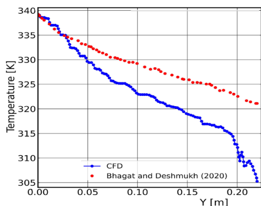
شکل ۱۸- نمودار توزیع دما در طول لوله ۵
