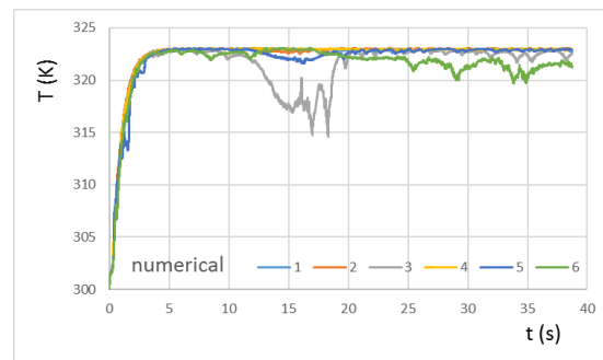
شکل ۱۹- دمای نقطه‌های ۱ تا ۶ بر حسب زمان
