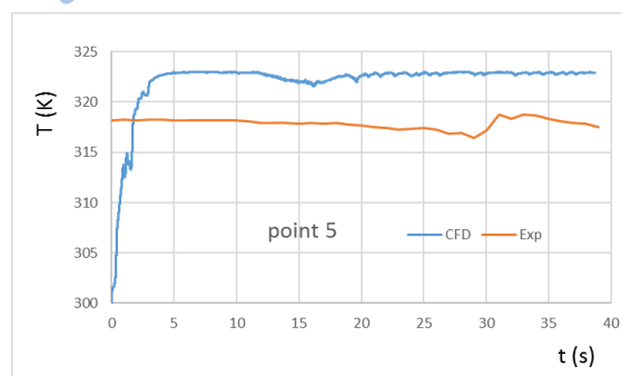
شکل ۲۱- دمای نقطه ۵ بر حسب زمان برای نتایج تجربی و عملی
