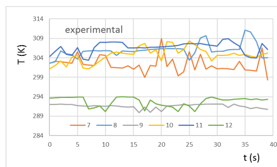
شکل ۱۳- دمای نقاط ۷ تا ۱۲ بر حسب زمان
