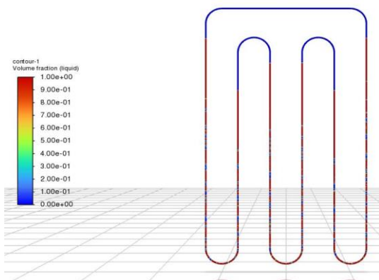
شکل ۲۴- کانتور کسر حجمی فاز مایع در زمان ۲۵/۹۱۵ ثانیه
