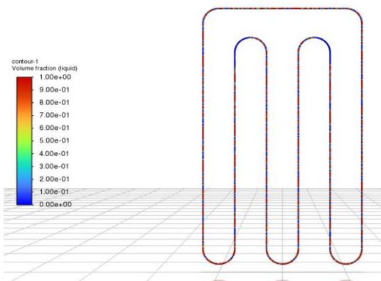
شکل ۲۵- کانتور کسر حجمی فاز مایع در زمان ۳۸/۷۱۳۵ ثانیه
