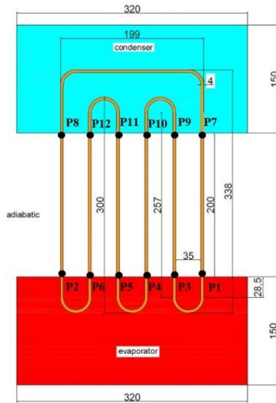
شکل ۴- ابعاد لوله گرمائی نوسانی حلقه بسته برحسب mm
