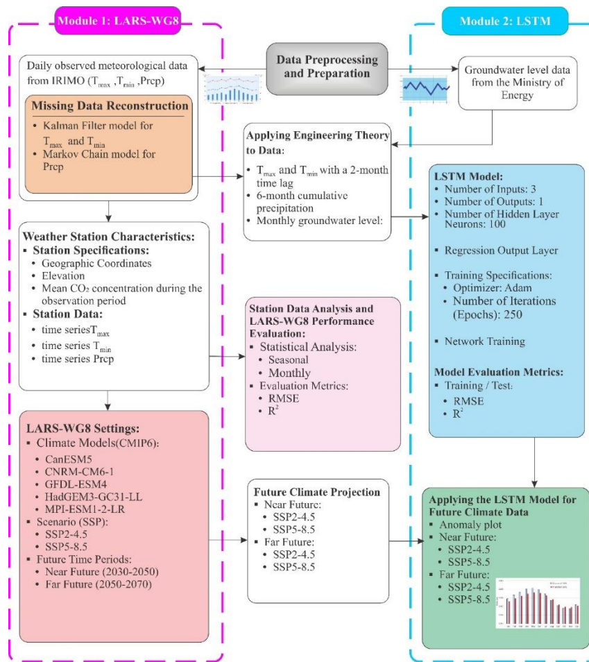
شکل ۲- فلوچارت روش شناسی. Figure 2- Methodological flowchart.
