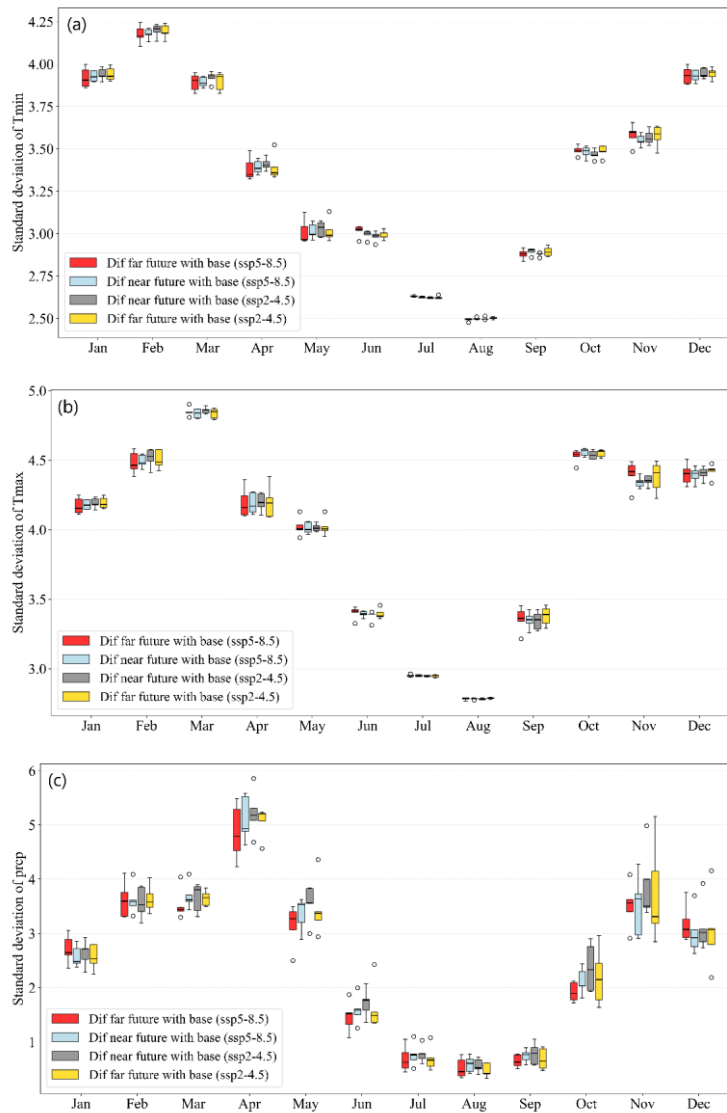
شکل ۵- نمودارهای جعبه‌ای ارزیابی عدم قطعیت: (الف) دمای حداقل، (ب) دمای حداکثر، (ج) بارش. Figure 5- Box plots for uncertainty assessment: (a) T_{min} ; (b) T_{max} ; (c) Precp.
