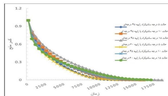
شکل ۱۴- تغییرات کسر مایع و روند انجماد برای دو زاویه اریب ۴۵ و ۶۰ درجه با دماهای متفاوت سیال انتقال گرما (۵، ۱۰، ۱۵ درجه سلسیوس)
