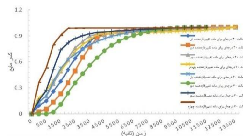
شکل ۲۰- تغییرات مایع در مبادله کن گرمایی با زاویه اریب ۳۰ و ۶۰ درجه با استفاده از انواع مواد تغییر فاز دهنده (ساده و چندگانه)
