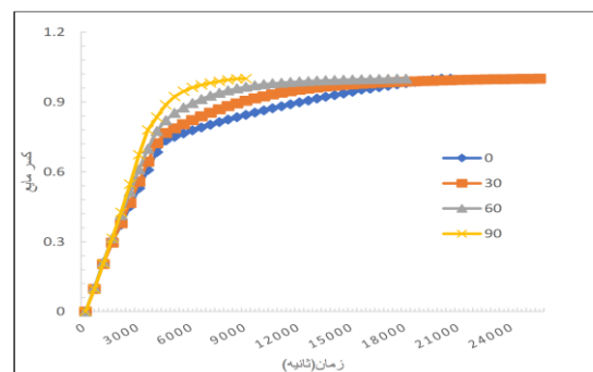
شکل ۱۷- تغییرات کسر مایع در فرایند ذوب برای قرارگیری مبادله‌کن گرمایی تک دوزنقه ای با زوایای ۰، ۳۰، ۶۰ و ۹۰ درجه ای نسبت به راستای افق دارای زاویه اریب ۶۰ درجه صفحات کانال
