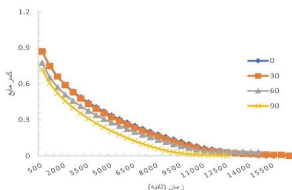
شکل ۱۸- تابع کسر مایع برای فرایند انجماد برای حالت زاویه انحراف مبادله‌کن گرمایی ۰، ۳۰، ۶۰ و ۹۰ درجه برای زاویه زیگزگ ۶۰ درجه
