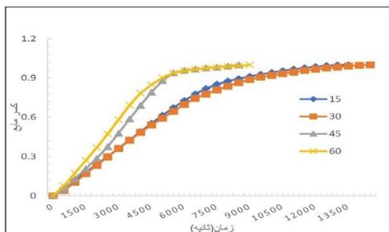
شکل ۸- تغییرات کسر مایع و روند ذوب برای چهار زاویه اریب ۳۰، ۴۵ و ۶۰ درجه
