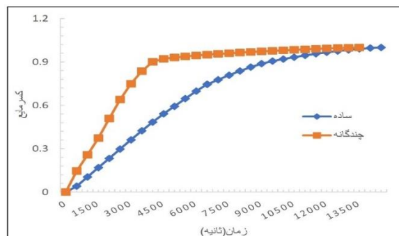
شکل ۱۹- تغییرات کسر مایع در یک مبادله کن گرمایی با زاویه اریب ۳۰ درجه با مواد تغییر فاز دهنده متفاوت (ساده و چندگانه)
