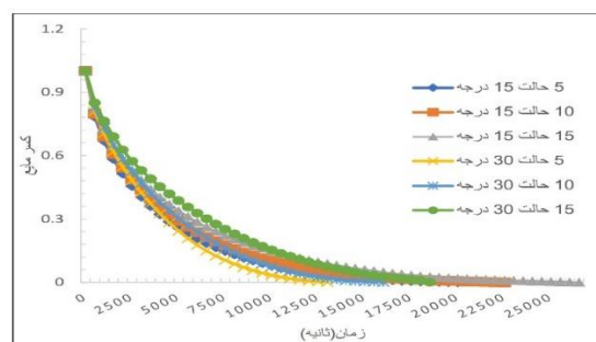
شکل ۱۳- تغییرات کسر مایع و روند انجماد برای دو زاویه اریب ۱۵ و ۳۰ درجه با دماهای متفاوت سیال انتقال گرما (۵، ۱۰، ۱۵ درجه سلسیوس)
