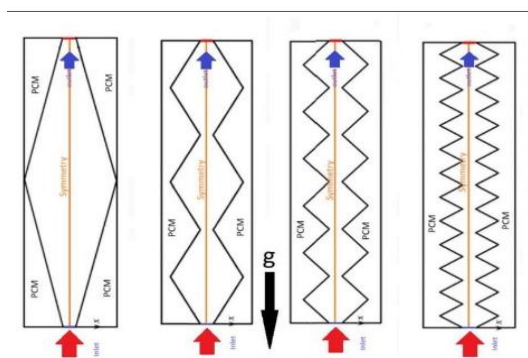
شکل ۱- مبادله‌کن گرمایی با صفحات کانال دارای زوایای اریب مختلف در مطالعه حاضر از راست به چپ به ترتیب 15^\circ ، 30^\circ ، 45^\circ و 60^\circ درجه
