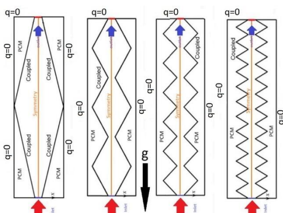
شکل ۲- شرایط مرزی حاکم (استفاده شده) برای سیال انتقال گرما و مواد تغییر فاز دهنده
