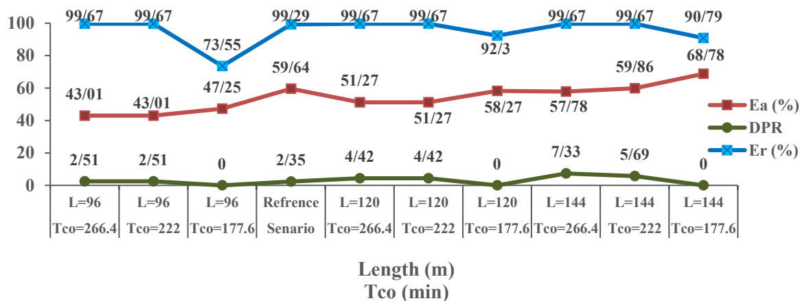
شکل ۸- تأثیر افزایش ۲۰ درصدی دبی ورودی و تغییرات طول جویچه و زمان قطع جریان بر پارامترهای DPR، Er و Ea
