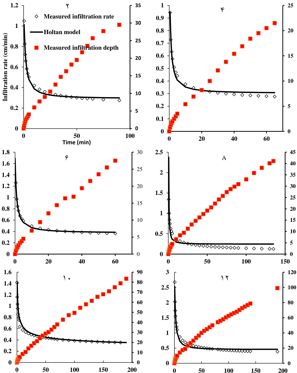
شکل ۲- منحنی نفوذ تجمعی اندازه‌گیری شده (نقاط مربع توپر) و شدت نفوذ محاسبه شده (نقاط لوزی توخالی) و برازش مدل هولتان بر داده‌های شدت نفوذ (خط پیوسته سیاه) در خاک ۶ از خاک ۱۲ مورد آزمایش. عدد بالای هر شکل بیانگر شماره نقطه مورد مطالعه در طول توپو سکانس است. محور عمودی سمت راست و چپ به ترتیب مقدار نفوذ تجمعی و سرعت نفوذ را نشان می‌دهند. منحنی نفوذ ۶ از خاک ۱۲ مورد آزمایش نشان داده نشده است.
