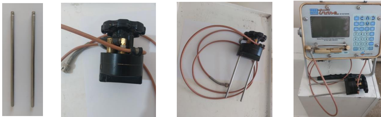
شکل ۱- به‌ترتیب از چپ به راست: میله‌های موج‌بر حسگر رطوبتی، کلاهک رابط، میله‌های موج‌بر همراه با کلاهک و سیم رابط و دستگاه TDR.
