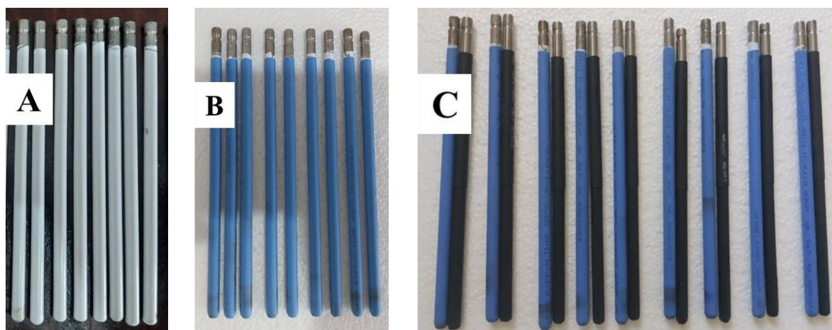
شکل ۴- حسگرهای رطوبتی تماسی رنگ‌آمیزی شده با رنگ سفید کوره‌ای (A)، حسگرهای رطوبتی تماسی رنگ‌آمیزی شده با رنگ سفید کوره‌ای با یک لایه پوشش شرینگ آبی رنگ (B) حسگر رطوبتی با ۲/۵ لایه پوشش شرینگ مشکی همراه با حسگرهای با پوشش رنگ کوره و شرینگ (C).
