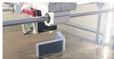
شکل ۷- چاپ قطعه نمونه در حالت خوابیده (سه‌محور)
