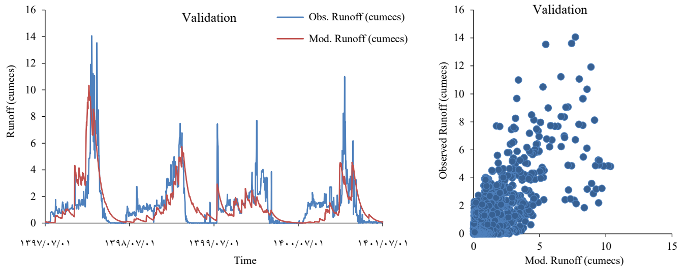
شکل ۵- سری زمانی و پراکنش رواناب مشاهداتی و شبیه‌سازی شده با مدل IHACRES در دوره‌های واسنجی و صحت‌سنجی.
