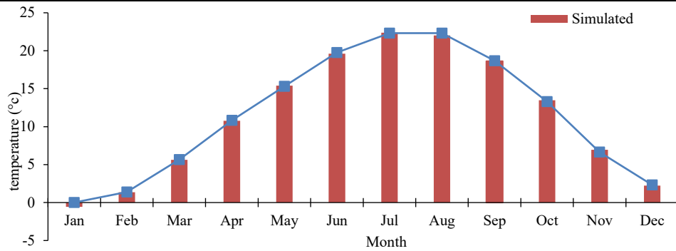
شکل ۳- مقایسه دمای میانگین مشاهداتی و شبیه‌سازی‌شده با استفاده از مدل لارس.
