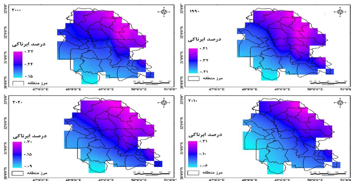
شکل ۳. توزیع فضایی درصد ابرناکی آسمان بر اثر ابرهای سطح میانی در فصل زمستان (میانگین ماه‌های ژانویه تا مارس) طی ۴ دوره آماری ۱۹۹۰-۲۰۲۰
