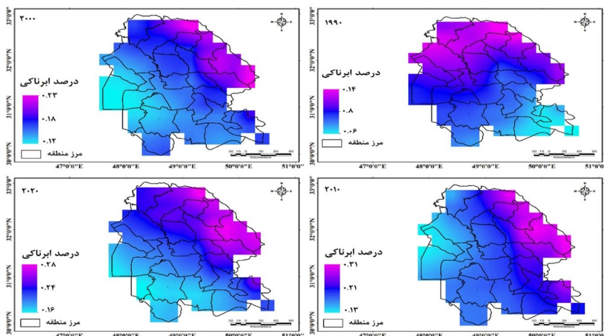
شکل ۵. توزیع فضایی درصد ابرناکی آسمان بر اثر ابرهای سطح میانی در فصل پاییز (میانگین ماه‌های اکتبر تا نوامبر) طی ۴ دوره آماری ۱۹۹۰-۲۰۲۰
