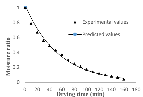
شکل ۶- تأیید مدل پیج اصلاح شده Fig. 6 Confirmation of modified Page model
