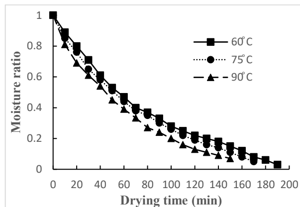
شکل ۳- نسبت رطوبت در مقابل زمان خشک شدن ورقه‌های پرتقال در دماهای مختلف (ضخامت ۶ میلی‌متر)
