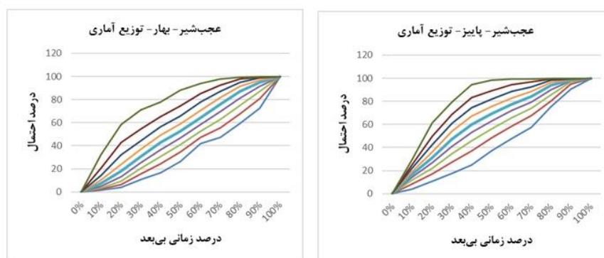
شکل ۵. منحنی‌های هاف تئوری برای ایستگاه عجشبیر در پاییز (راست) و بهار (چپ) حاصل از برازش توزیع‌های آماری
