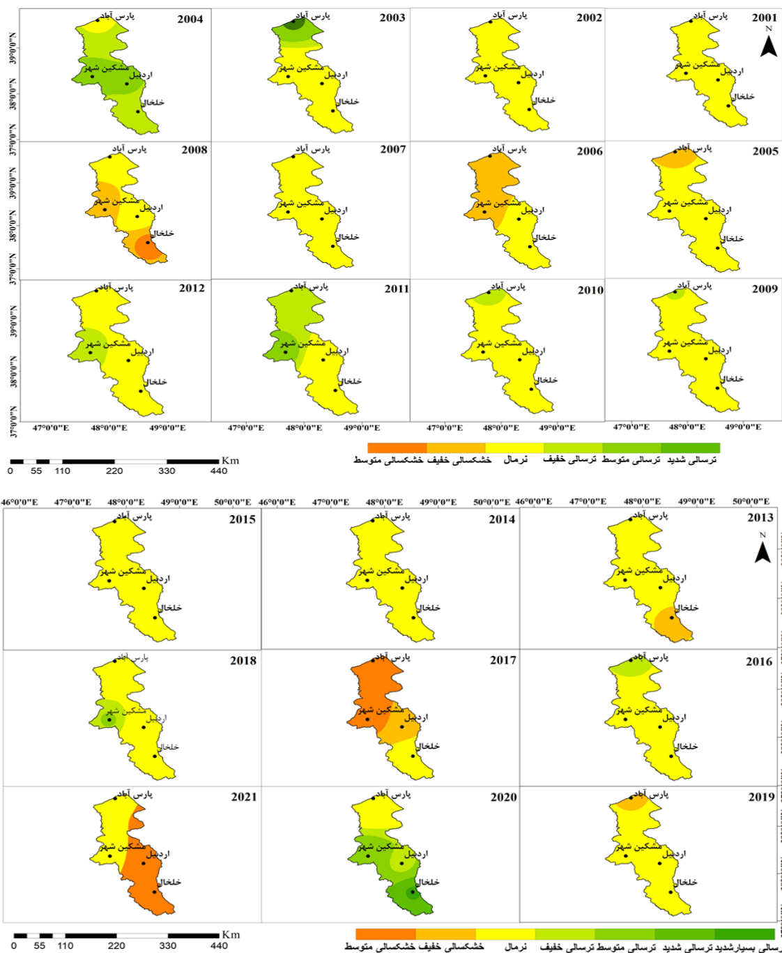
شکل ۶. بررسی خشک‌سالی براساس کلاس‌بندی سری زمانی مقادیر PNPI طی سال‌های ۲۰۰۱ تا ۲۰۲۱ (منبع: یافته‌های تحقیق)
