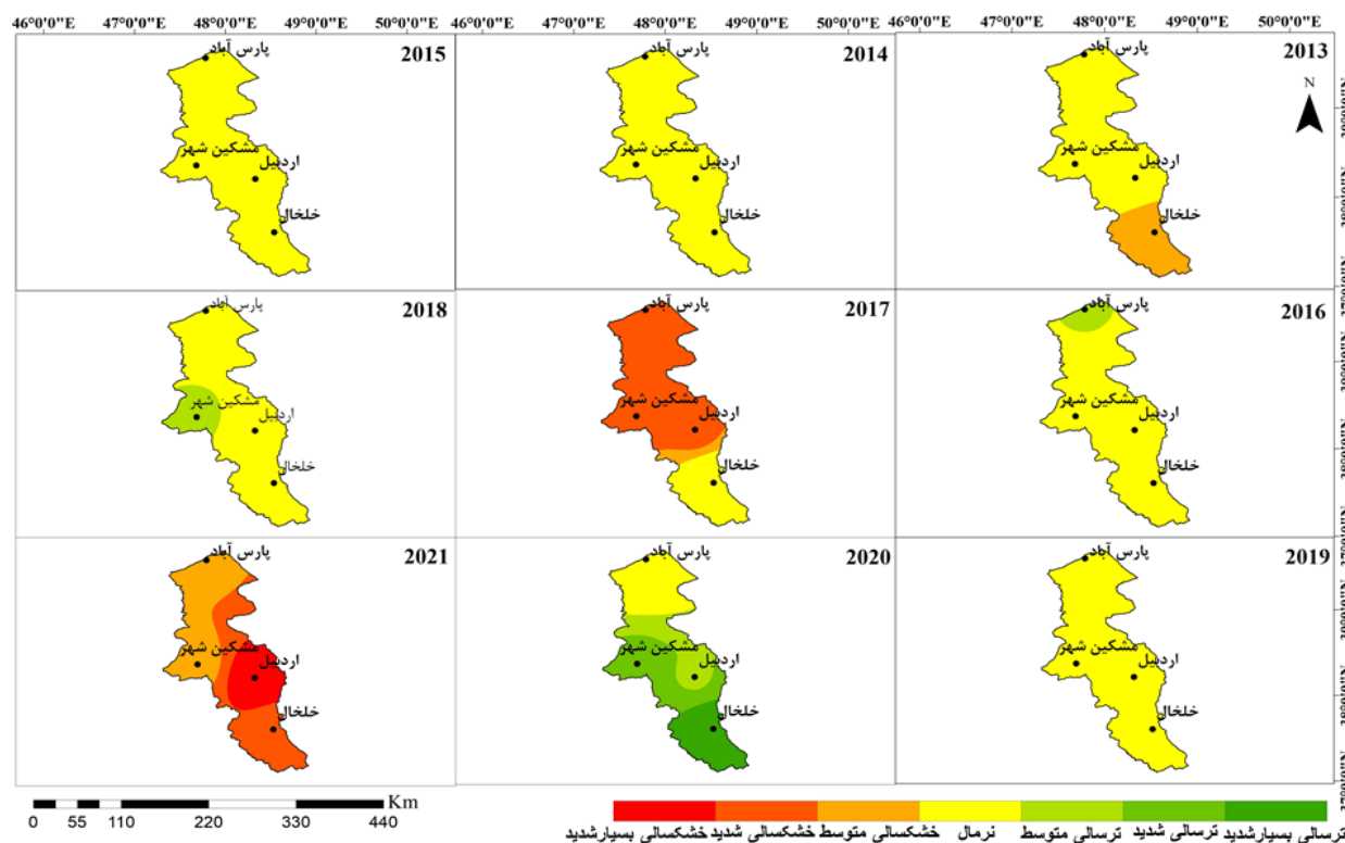
شکل ۳. بررسی خشک سالی براساس کلاس بندی سری زمانی مقادیر SPI طی سالهای ۲۰۰۱ تا ۲۰۲۱ (منبع: یافته‌های تحقیق)
