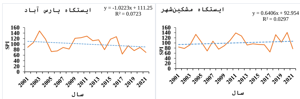
شکل ۴. نمودار روند مقادیر شاخص PNPI برای ایستگاه‌های مورد مطالعه طی دوره آماری (۲۰۰۱-۲۰۲۱) (منبع: یافته‌های تحقیق)
