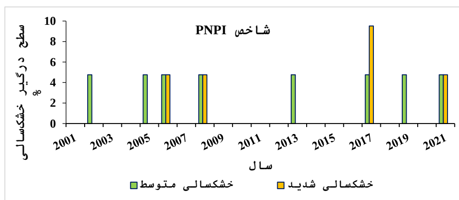
شکل ۷. سطوح درگیر خشکسالی در استان اردبیل طی دوره آماری (۲۰۲۱-۲۰۰۱) با استفاده از شاخص‌های SPI و PNPI (منبع: یافته‌های تحقیق)
