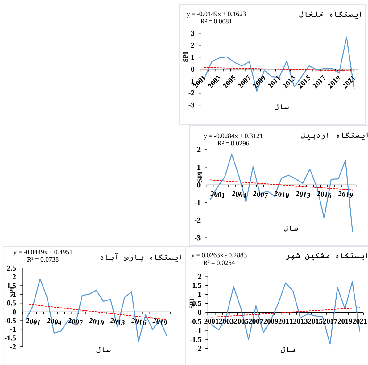
شکل ۲. شاخص بارش استاندارد (SPI) در ایستگاه‌های مورد مطالعه در طول دوره آماری (۲۰۰۱-۲۰۲۱) (منبع: یافته‌های تحقیق)
