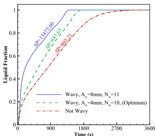
شکل ۷- تغییرات زمانی میانگین کسر مایع در مبادله‌کن گرمایی با دیوارهای میانی مختلف
