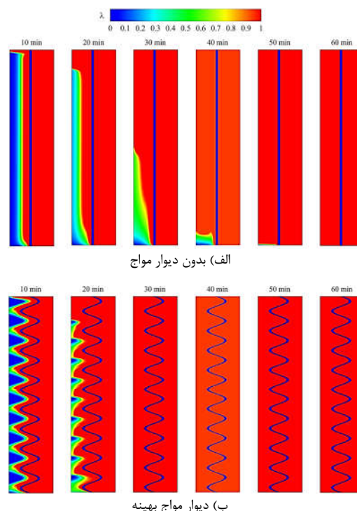
شکل ۶- کانتور تغییرات زمانی کسر مایع در سیستم ذخیره‌سازی (الف) بدون دیوار موج و (ب) با دیوار موج بهینه
