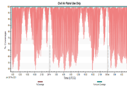
شکل ۳- پوشش‌دهی منظومه ۲۲۰ ماهواره‌ای Starlink برای کشور ایران
