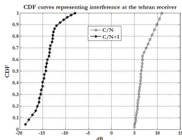
شکل ۷- میزان CDF توابع C/N+I و C/N در سناریوی تداخل DL
