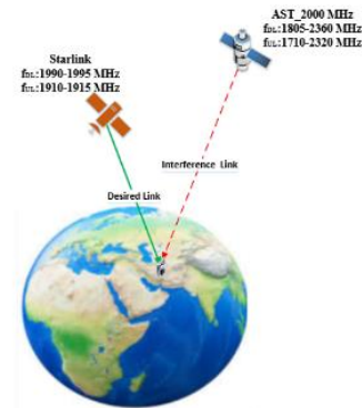
شکل ۶- نحوه تداخل ماهواره AST 2000 MHz در مسیر DL بر روی لینک ایجاد شده مابین گوشی کاربر زمینی و ماهواره Starlink
