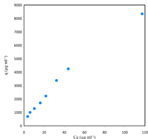
شکل ۳- همدمای جذب سطحی تولوئن در سیستم هیومین-تولوئن.
