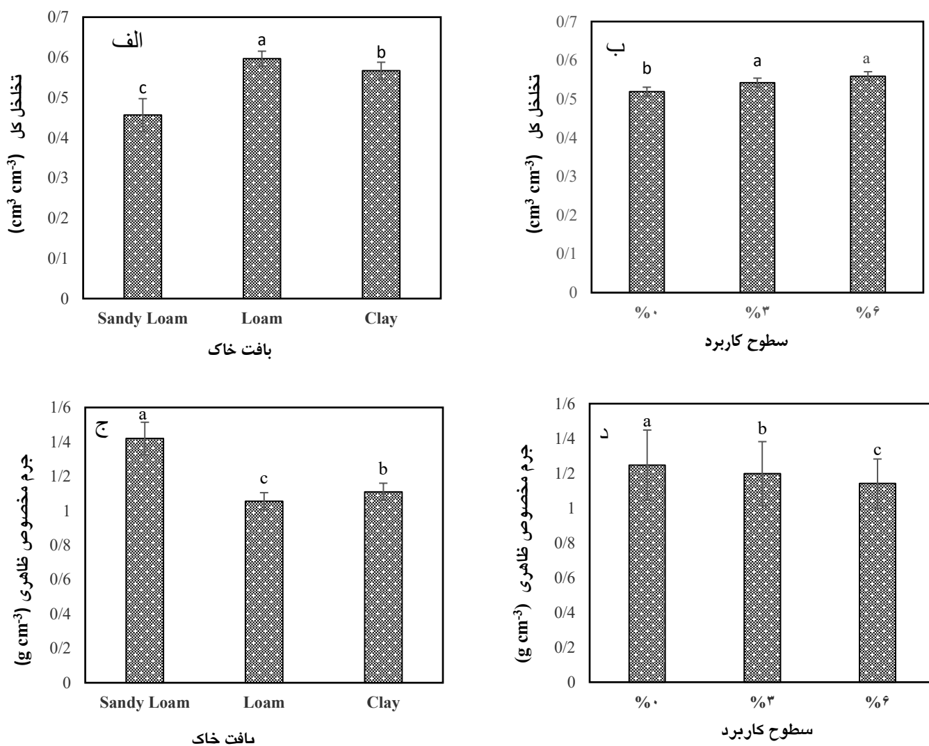
شکل ۲- اثر اصلی بافت خاک (الف و ج) و سطوح کاربرد کمپوست بستر قارچ (ب و د) به ترتیب بر تخلخل کل و جرم مخصوص ظاهری خاک. در هر شکل وجود حروف مشابه بر روی هر یک از ستون‌ها نشان‌دهنده عدم وجود تفاوت معنی‌دار در سطح ۵ درصد آزمون دانکن می‌باشد. خطوط عمودی بر روی هر ستون نشان‌دهنده انحراف استاندارد داده‌ها است.
