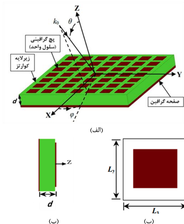
شکل ۱۲- (الف) نمای کلی از ساختار متناوب جاذب، (ب) دید از بالای سلول واحد با پچ گرافینی، و (پ) دید از پهلوی سلول واحد با ضخامت زیرلایه d .
