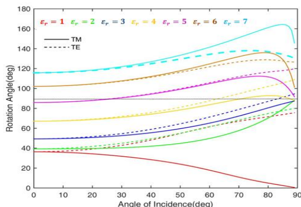
شکل ۱۴- زاویه چرخش برحسب زاویه تابش برای عایق‌های مختلف ساندویچ شده بین صفحات گرافین، در بایاس مغناطیسی B_0=1T (f=30\text{GHz}, \mu_c=0.37\text{eV}, \tau=1.84 \times 10^{-13}\text{s}, n_s=10^{13}\text{cm}^{-2}, d=2\text{mm}, T=300K)
