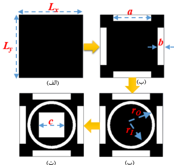
شکل ۱۴- مراحل رسیدن به پچ گرافینی در سلول واحد جذب
