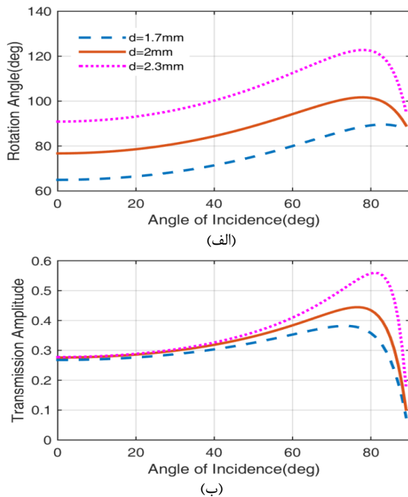
شکل ۴- (الف) زاویه چرخش بر حسب زاویه تابش و (ب) دامنه انتقال بر حسب زاویه تابش، هردو با تغییرات ضخامت لایه میانی کوارتز و در قطبش TM ( B_0=1T , f=30\text{GHz} , \epsilon_r=3.82 ). مقادیر ارائه شده d در (الف) با همان شکل و رنگ نمودار برای شکل (ب) نیز برقرار است.
