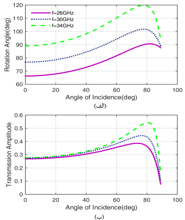
شکل ۵- (الف) زاویه چرخش برحسب زاویه تابش و (ب) دامنه انتقال برحسب زاویه تابش، هردو با تغییرات فرکانس و در قطبش TM ( B_0 = 1\text{T} , d = 2\text{mm} , \epsilon_r = 3.82 ) در (الف) با همان شکل و رنگ نمودار برای شکل (ب) نیز برقرار است.
