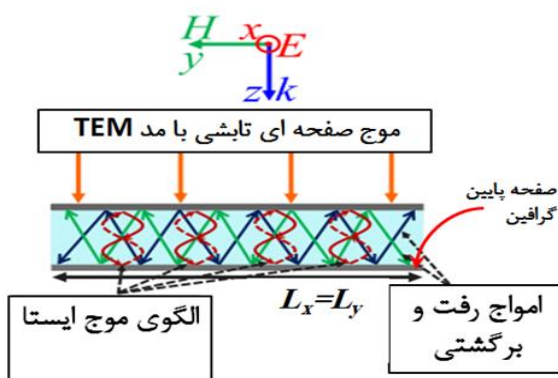
شکل ۱۶- مدل موج ایستای ایجاد شونده داخل سلول واحد جذب و نقش صفحه پایینی گرافین در وقوع چنین پدیده‌ای.
