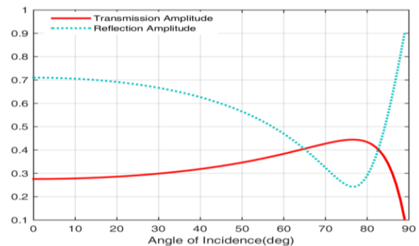
شکل ۳- اندازه ضرایب انتقال و بازتاب بر حسب زاویه تابش برای ساختار گرافین-کوارتز-گرافین تحت بایاس مغناطیسی B_0=1T و قطبش TM ( \tau=1.84 \times 10^{-13}s , n_s=10^{13}cm^{-2} , \epsilon_r=3.82 , \mu_c=0.37eV , d=2mm , T=300K , f=30GHz ).
