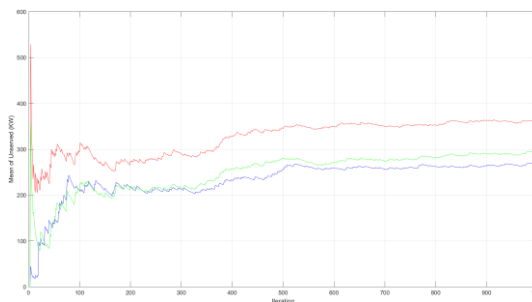
شکل ۳- بار ازدست رفته در شبکه اصلی (نمودار قرمز)، شبکه بازآرایی شده توسط روش مقاله [۲۱] (نمودار سبز) و شبکه بازآرایی شده توسط روش پیشنهادی (نمودار آبی)
