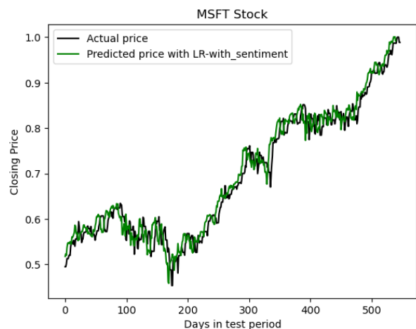
شکل ۹- پیش‌بینی سهام توسط روش LR با تحلیل احساسات
