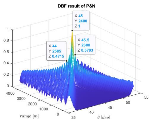
شکل ۵- تزویج بین (R, \theta) در کد فرکانسی ترتیبی مثبت و منفی
