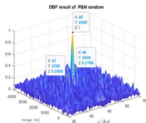
شکل ۱۱- تزویج بین (R, \varphi) در کد فرکانسی پیشنهادی
