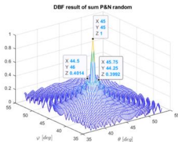
شکل ۱۲- تزویج بین (\theta, \varphi) برای تمام کدهای فرکانسی
