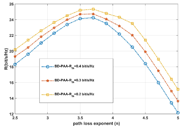
شکل ۶- تغییرات مجموع گذردهی کاربران بر حسب تغییرات نمای
