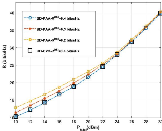
شکل ۵- تغییرات مجموع گذردهای کاربران بر حسب تغییرات توان کل برای حداقل گذردهای تضمین شده مختلف برای کاربران
