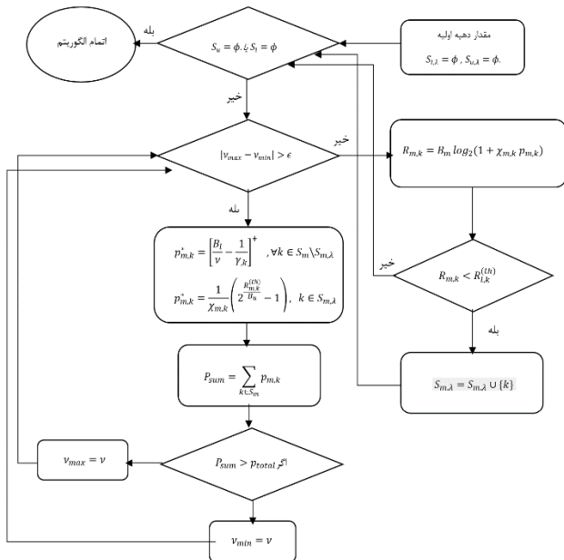
شکل ۲- فلوچارت الگوریتم تخصیص توان پیشنهادی
