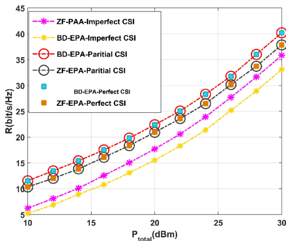
شکل ۷- تغییرات مجموع گذردهی کاربران بر حسب تغییرات توان کل تحت فرض‌های CSI کامل و ناقص
