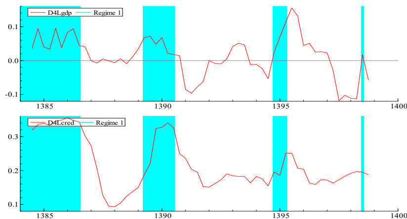
نمودار (۲): تفکیک رژیم‌ها بر اساس احتمالات هموارشده ۱
