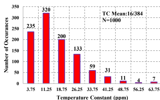
شکل ۱۶: نمودار هیستوگرام ضریب تغییرات دمایی به ازای ۱۰۰۰ بار تکرار در شبیه‌سازی مونت کارلو
