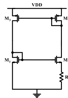
شکل ۲: مرجع جریان PTAT با ترانزیستورهای زیر آستانه
