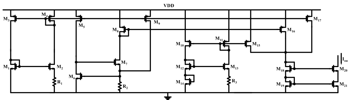
شکل ۷: ساختار مداری مرجع جریان پیشنهادی
