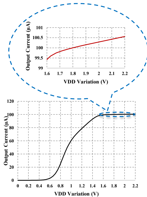
شکل ۱۰: نمودار جریان خروجی بر حسب تغییرات تغذیه
