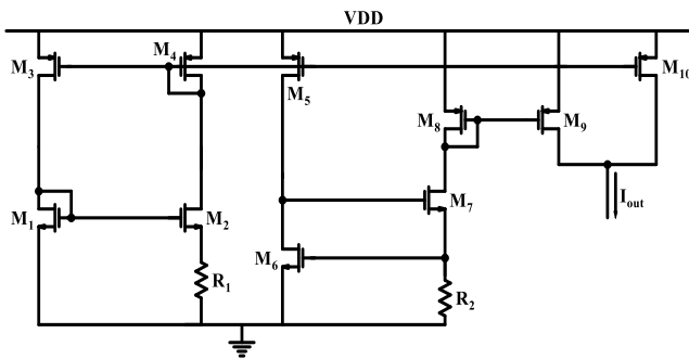
شکل ۳: ترکیب جریان های CTAT و PTAT ترانزیستورهای زیر آستانه
