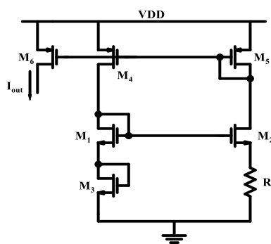
شکل ۵: مرجع جریان با ترانزیستورهای ناحیه اشباع [۶]
