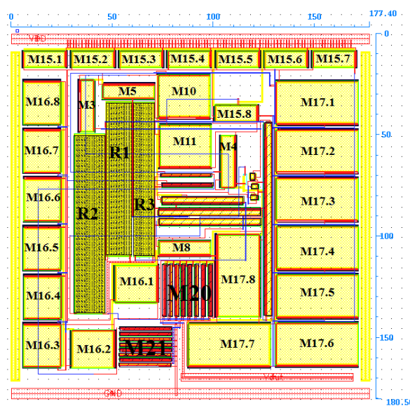
شکل ۸: طرح جانمایی مدار پیشنهادی
