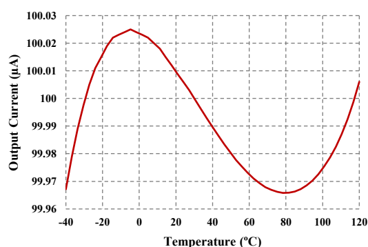
شکل ۹: جریان خروجی در محدوده دمایی -40^{\circ}C تا 120^{\circ}C
