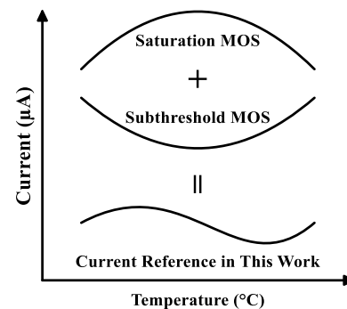
شکل ۶: ترکیب ساختار ترانزیستورهای زیرآستانه و اشباع
